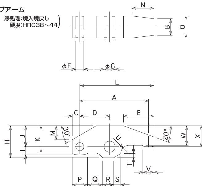
寸法表
