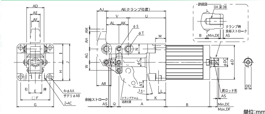
JLF5H形 配管口位置めねじ配管 (K) 寸法図
