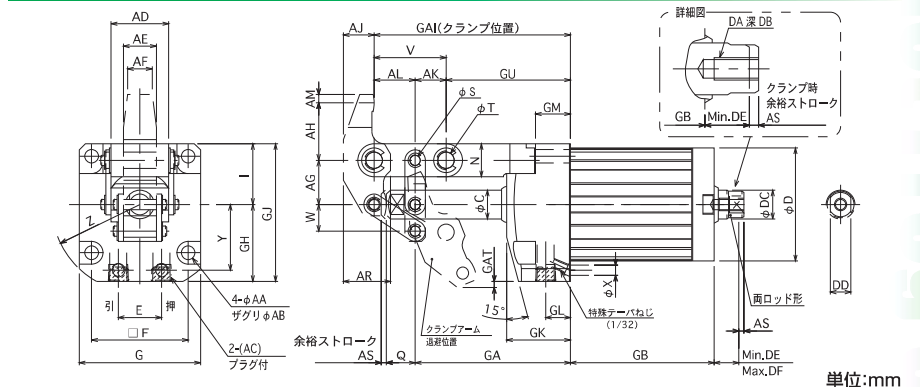
JLF5H形 配管口位置ガスケット配管 (G) 寸法図
