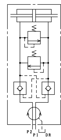
油圧回路図
