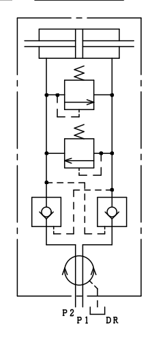
油圧回路図
