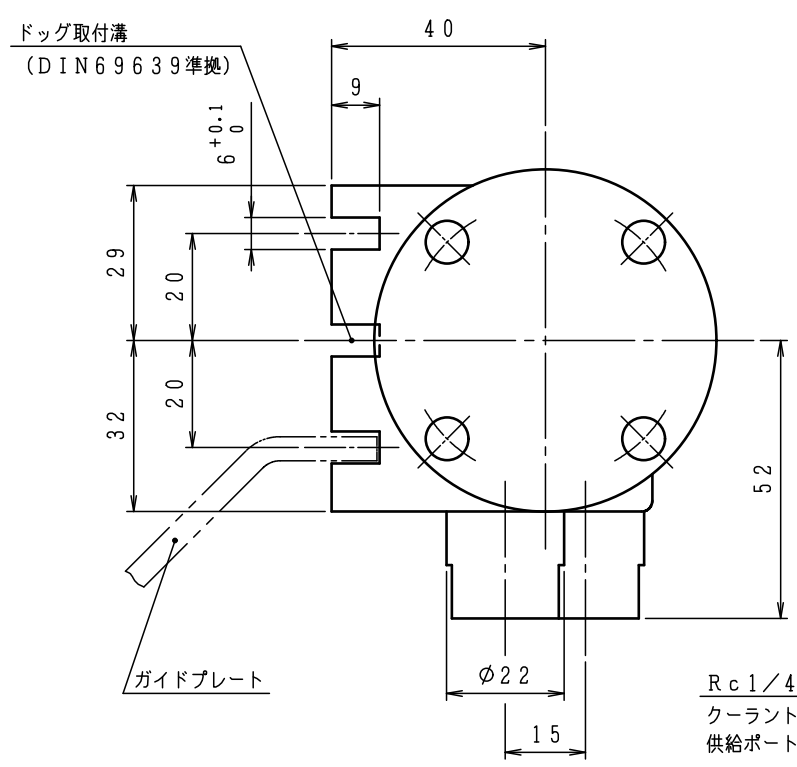
回転継手シール面潤滑方法の例
