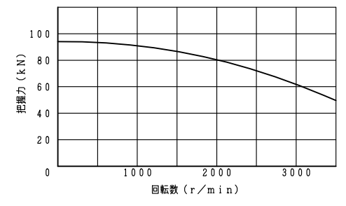
把握力特性図 (標準生爪使用時)
