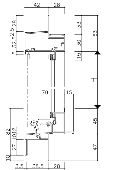
< 鉄骨半外付 >
