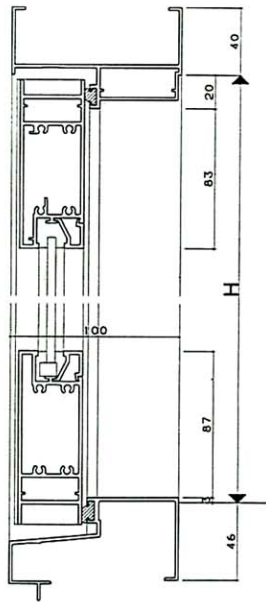
〈ガラス溝 15 〉
