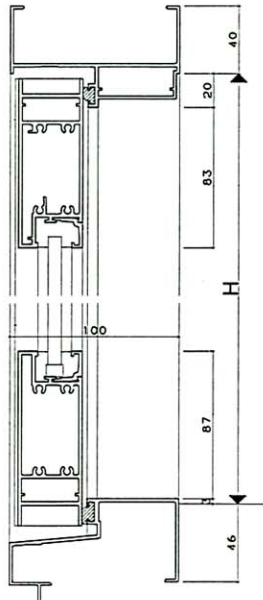
〈ガラス溝 20 〉
