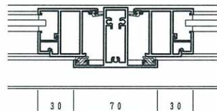
方立部
