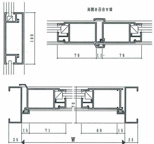
中框
