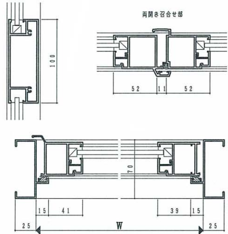
中框
