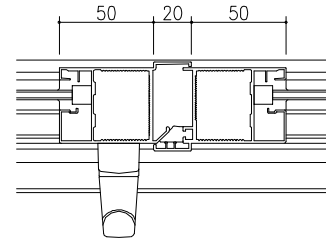
< 袖FIX部 >
