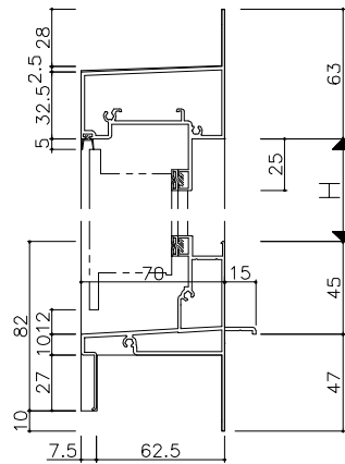
< 鉄骨外付 >
