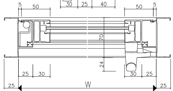
< 鉄骨半外付 >
