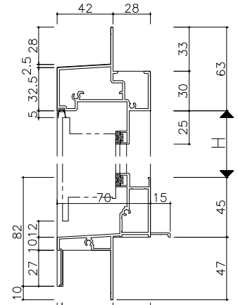
< 鉄骨半外付 >
