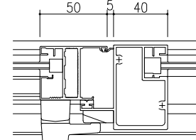
< 袖FIX部 >
