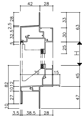
< 鉄骨半外付 >
